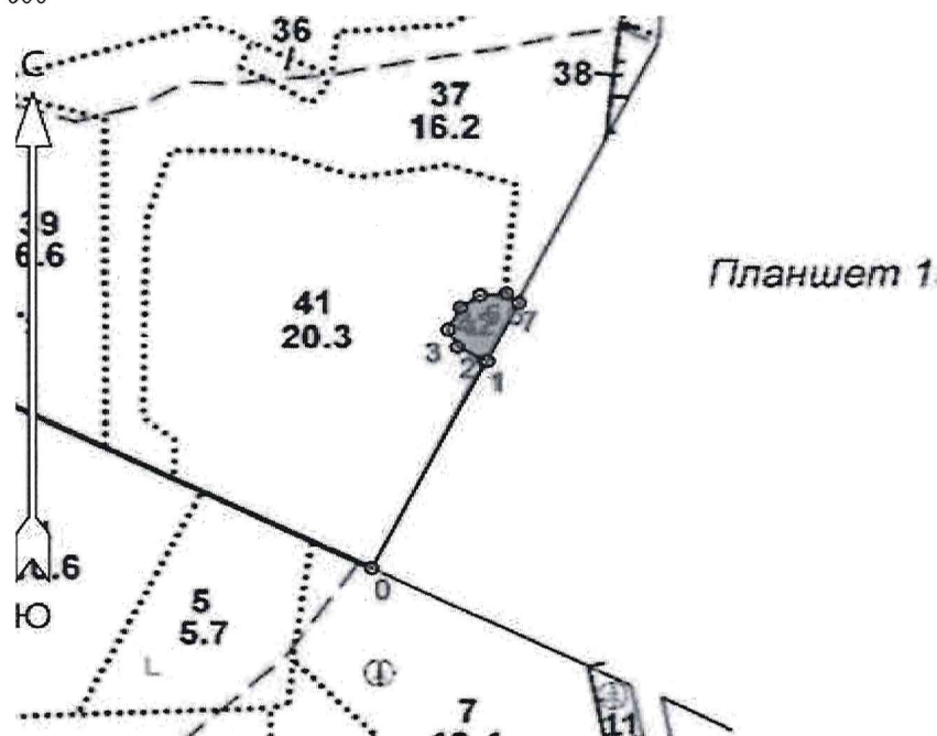
Экспликация участка
