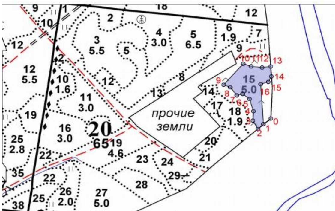
Экспликация участка
